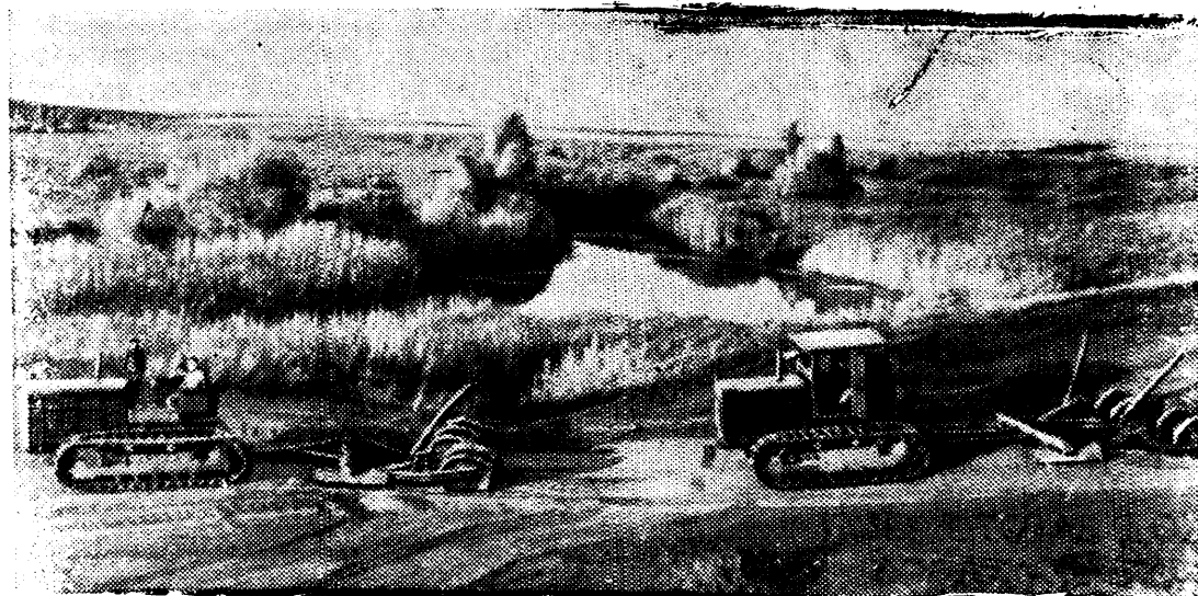
ЧКАЛОВСКАЯ ОБЛАСТЬ. Колхоз имени Чапаева Илекского района строит на реке Заживная плотину шириной 450 метров и высотой 10,5 метра.
