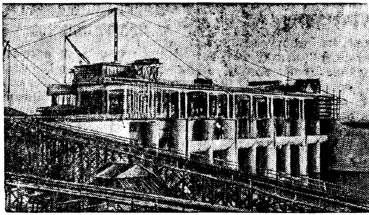
Общий вид железобетонной плотины № 2 Фото М. Королева. Фото-книжка ТАСС.
