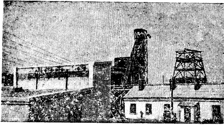
Общий вид строительства шахты № 24 треста Сталиногорскшахтстрой. В сентябре шахта вступила в строй действующих предприятий.
