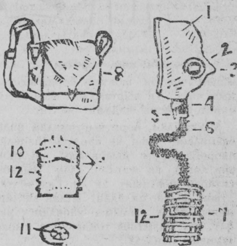
Рис. 3 Противогаз „Т.Т.С.“ 1-шлэм- маскы; 2—сйзйлык; 3-стьокла йштйлымь парняшка, 4-кым ыражан изи пыч (патрубок—тройник). 5-шүлым лыкмы йраж, 6-кукшы логер постол пыч, 7-йадан газым ирыктышы фильтр—коропля, 8-тйпняк, 9-рэшоткан кядэжвлэ, 10-тангыла пружина, 11-воздух пйртымь клапан пробка, 12-коропляштыш ладиквлэ (зигвлэ).
