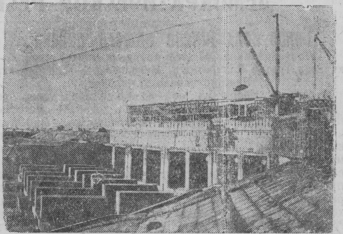
На снимке: Панорама строительства плотины № 2. (Вид с нижнего бьефа).
