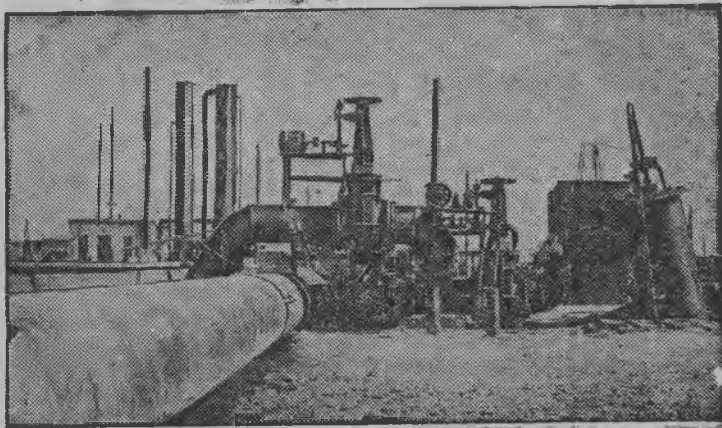
Суред вылын: Донбассын эгырлэн подземной газификациялэн первой станциясы.
