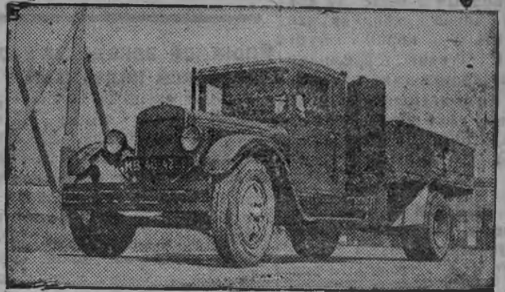
НАТИ-ын (научной авто-тракторной институт) сконструировать каремын грузовой трехтонной „ЗИС-5“ машиналы газогенераторной установка Г-23, куд'ёсыз ужало пу эгырен. Та машинаослэн эксплуатацизы кыкполэс дунтэм усе.
