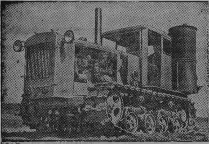
Суредын газогенераторной трактор ХТЗ.
