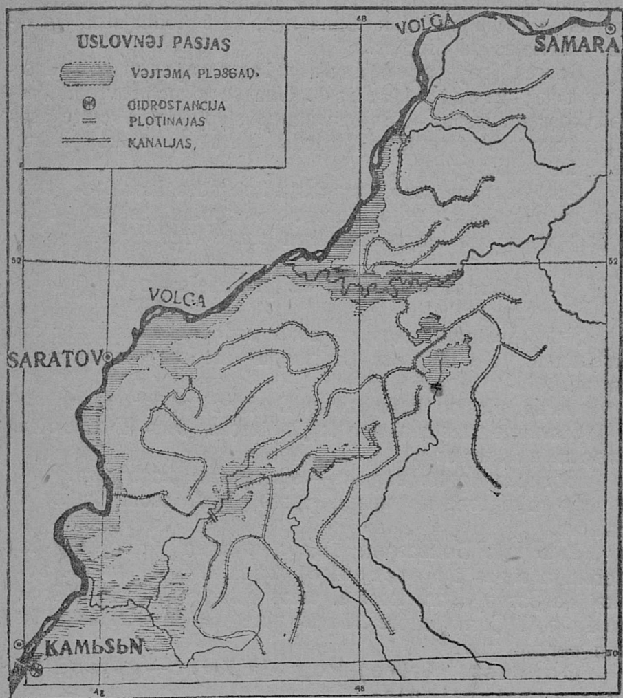
Niznej Zavolžjə orosajtan sxema.
