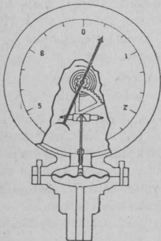
79 şer. Manometra.
