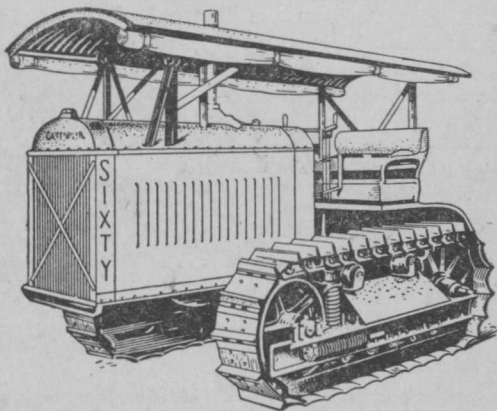
61 šer. Gušenicaa traktor.
