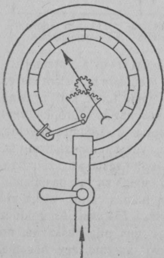
117 җәр. Manometra.
