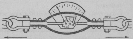
39 шер. Динамометра.
