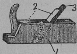
18 ris. Serxevel: 1 — kolodka, 2 — tuv, 3 — zelezko.
