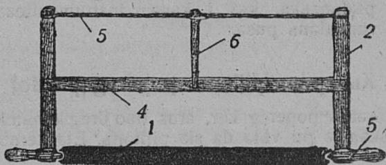
10. Луçковėj пилa: 1—лис, 2—орop (ручка), 3—сафовна, 4—распорка, 5—уттѣва, 6—закрутка.
