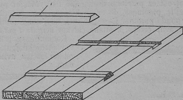
41 ris. Sponkaezән әтлаәтәм: 1 — sponka.
