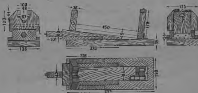
12-шы рис. Цельаш тымэньмаш станок.
