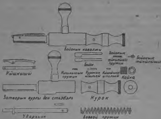
29-шы а рис. Затвор.
