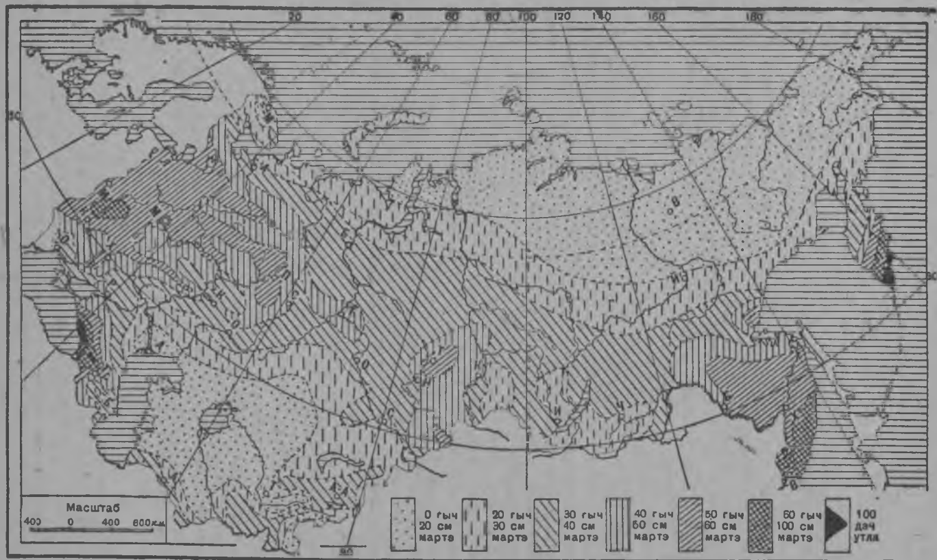
27 сур. Йуж-вуд идалык мучко монар вочым ончыктышо карт.
