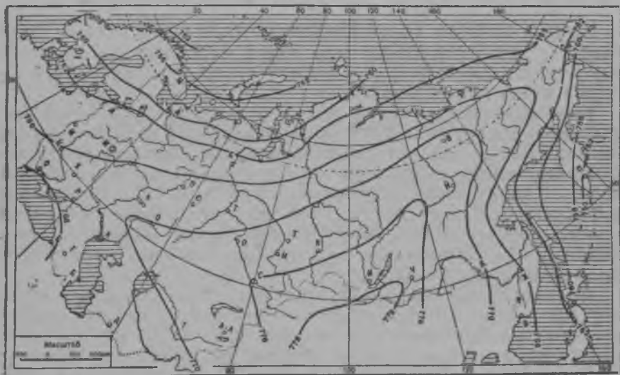
24 сүр. Йанвар тылээ изобар-влак.
