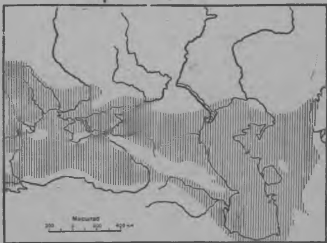
7 сур. Акрәт годсо Шәм тэнгыз-каспий басәйн. (Тэнгыз налмә вәрым штрихлән ончыктымә).
