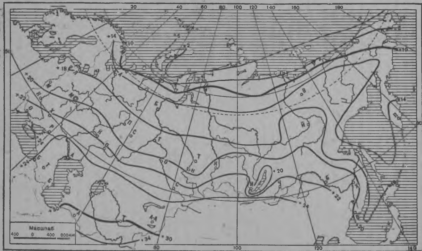
23 сур. Ийуль изотерм-влак
