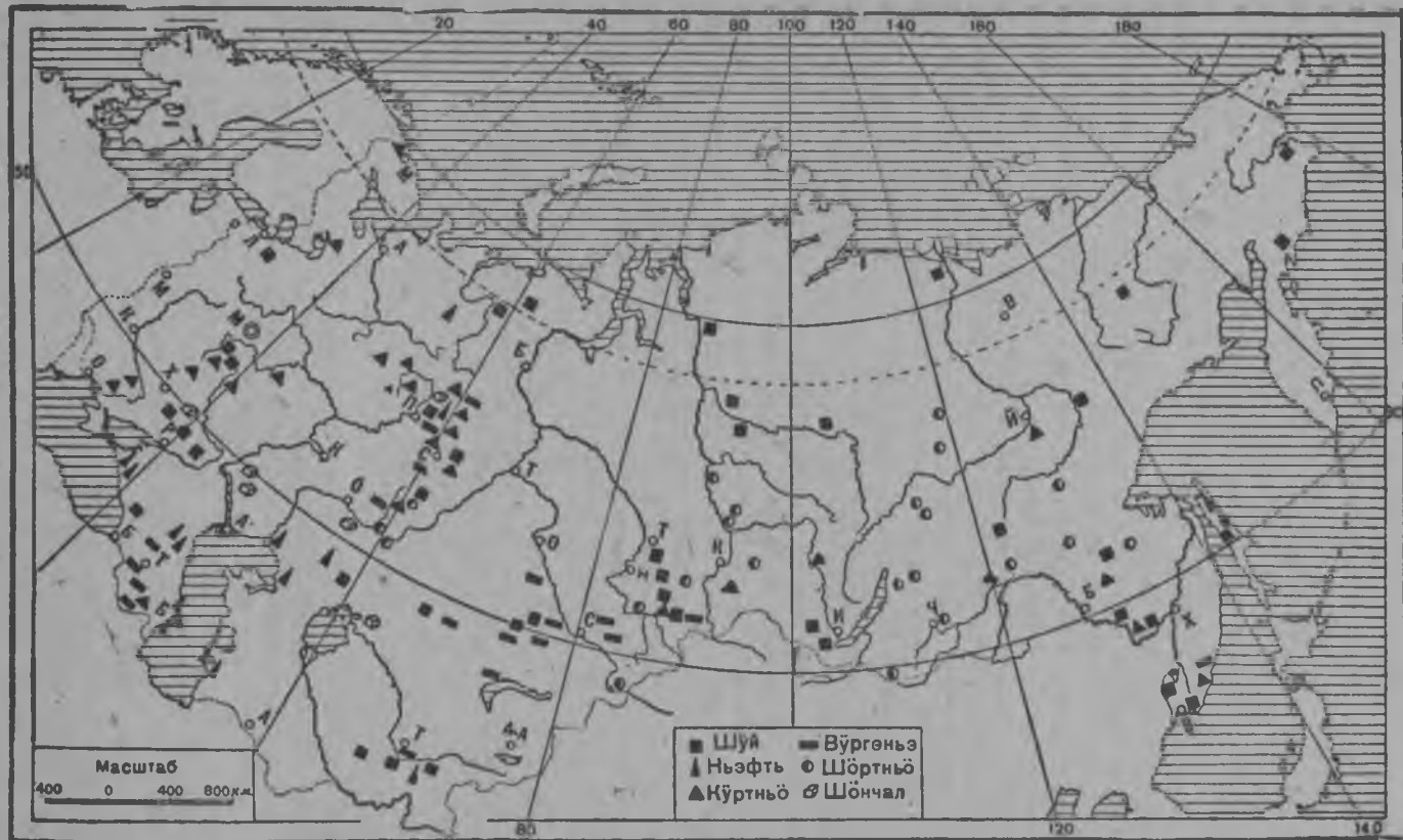
20 сүр. ССР Ушэмын күнчэн лукмо пойанлык кийымым ончыктышо карт.
