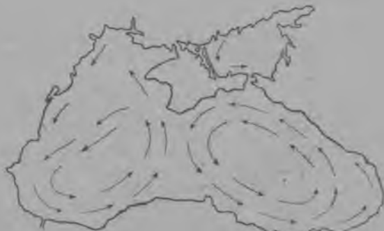
6 сўр. Шэм тэнгызысэ йогын-влак.
