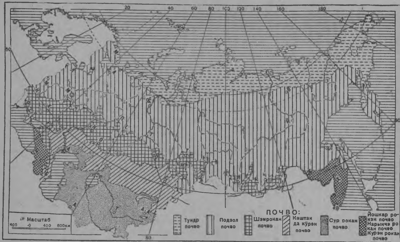
36 сўр. ССР Ушэмын почво картшэ,
