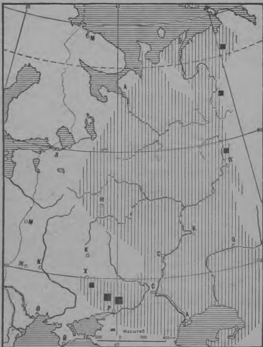
18 сүр. Эрвэйлэвроп төр вэрыштэ мландэ шүй лиймэ жапыштэ тэгыз шарлымэ вэр. (Штрихлэн тэгызым очныктымо, шэм квадрат-влак дэн — мландэ шүй кийымэ вэрым).
