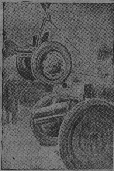
Отгрузка готовых орудий в одном из цехов Н-ского завода (Ленинград). Фото В. Федосеева.
