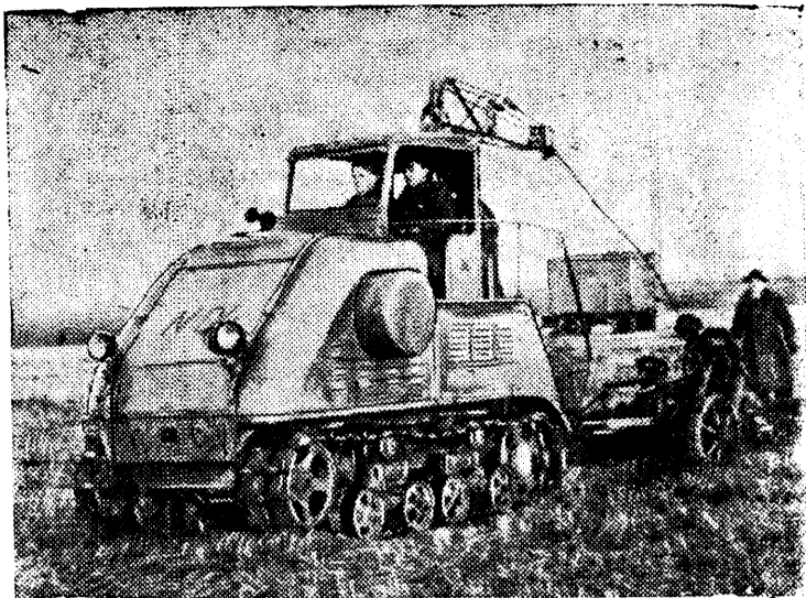
КИЕВСКАЯ ОБЛАСТЬ. В Корсунь-Шевченковском районе создана электромашинно-тракторная станция. На снимке: электротрактор поднимает пары на полях колхоза «Червона Рось». Фото М. Немеймана. Прессфото ТАСС.
