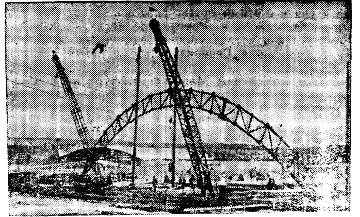
Установка первой арки на русловой площадке гидро-технической лаборатории. Фото Н. Славина. Фото-клише ТАСС.
