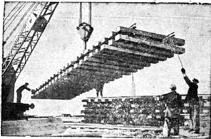
На снимке: Погрузка звеньев на платформы с помощью погрузочного крана—путькладчика для отправки к месту укладки пути. Фото А. Бахвалова. Бюро-клише ТАСС.
