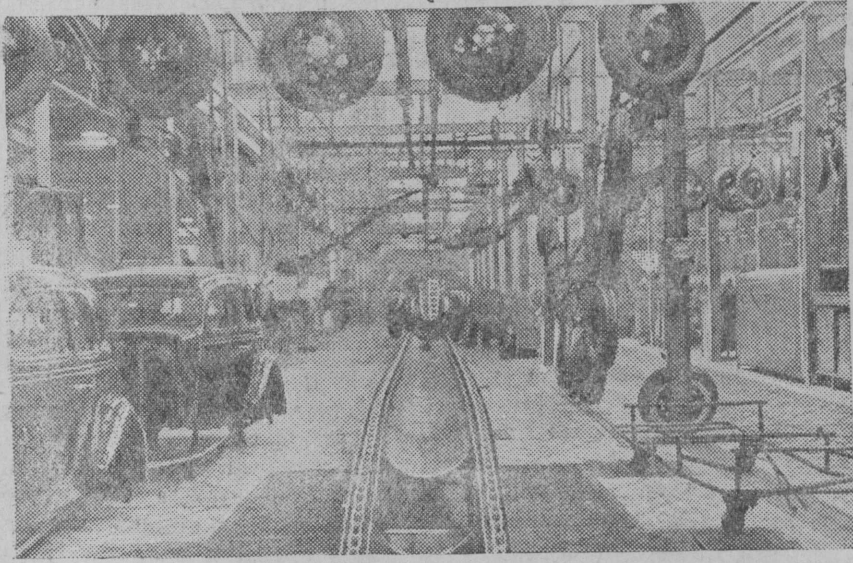
Московский завод им. Сталина. НА СНИМКЕ: главный конвейер легковых машин ЗИС-101.
