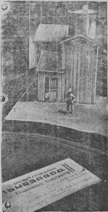
На областной выставке колхозного льноводства. Макет одноэтажного льнозавода Калининского льнотреста
