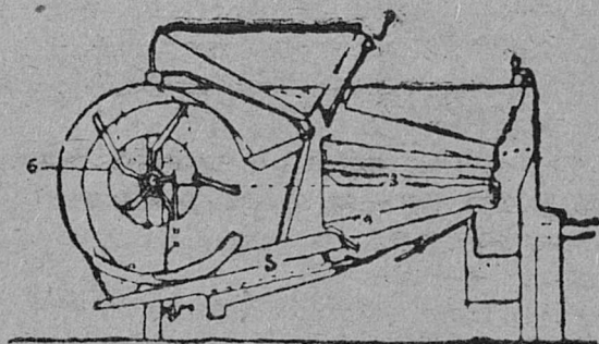
2-öd серпас. Клејтон типа 5-öd № вежалка-сортировкалөн пыщкөсыс (разрез).
