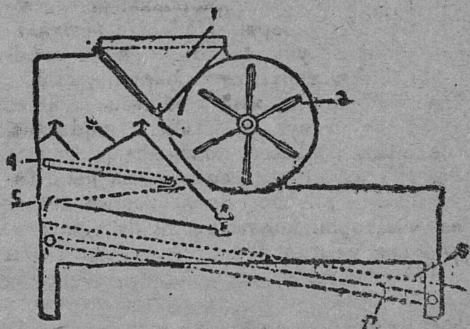
20-бд сөрпәс. „Кускута“ сортировкадн пыщкөсыс (схема). 1—күстәән көч, 2—вентиләтөр, 3—пыщкөсыс сәжд (щит), 4—вылыс пож, 5—мөд пож, 6—улыс куә пож, 7—улыс пож весәән щөткајас.
