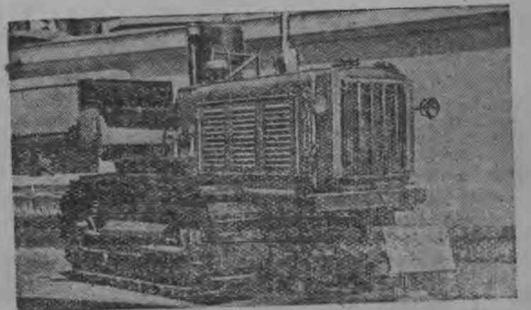
Новый экспонат павильона Механизации опытный образец гусеничного трактора ЧТЗ-Г-3465 с газогенераторной установкой НАТИ Г-34, работающий на древесном угле. Мощность двигателя 65 лошадиных сил. Фото С. Шагалъ. Фото-Клише ТАСС.
