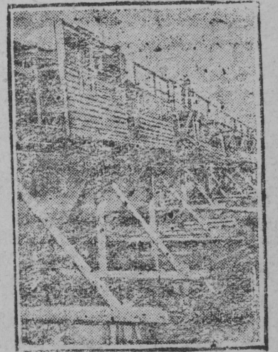
На снимке: Подвесная лесовозная дорога нового типа. Поезд груженный лесом идет по эстакаде под дорогом через реку Двиницу (Сев. край).
