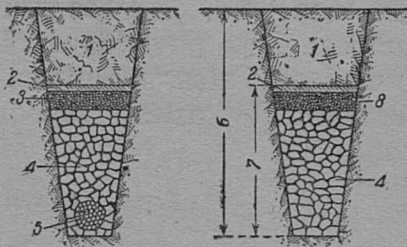
14 šerp. 1 — mu; 2 — eza; 3 — poŋi gałki; 4 — gałki livə iz torьrič; 5 — fasina 6 — 1—1,25 metrəz; 7 — \frac{2}{3} zusta; 8 — gьbš lьa.
