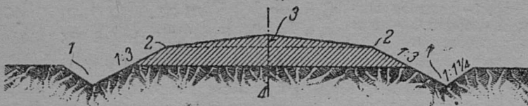
6 şəsr. 1—кјувет; 2—вропка; 3—вропкашаьс вьлпзк— 0,13—0,25 метр; 4—туј ош.
