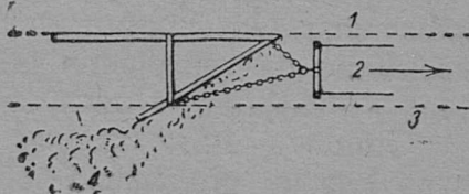
20 şerp. 1—kujim peļəsa kanavalən pьdəstiyş; 2—kodarə vəlyş munə; 3—tuj brovka; 4—kanavakodjanən sьvətəm grunt.
