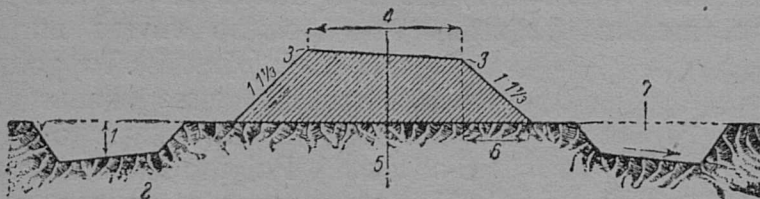
5 şəsr. 1—ауштаьс ипавьлә 1 м; 2—рәкат; 3—вропка; 4—ролотнолән раштаьс; 5—туј ош; 6—откос залозендә; 7—резерв.
