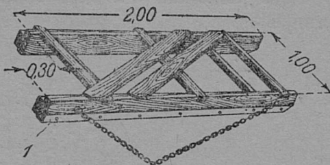
21 şerp. 1—kərt plankə 100×5 mm.
