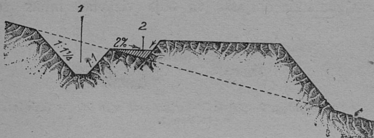
12 şərp. 1—nagornəj da vakьskəd kanava; 2—verma.
