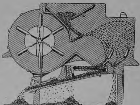
7-шы карт. Пьрць итьрājьымь машинāн ровотаймыжы.
