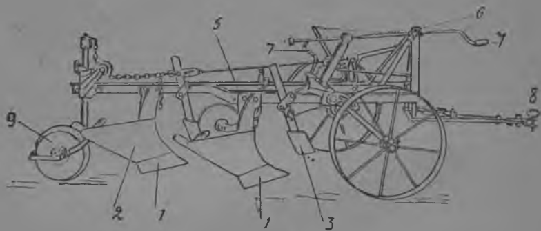
7-тй суред. Тракторен ужан плуг ожо кесянэн валче.
